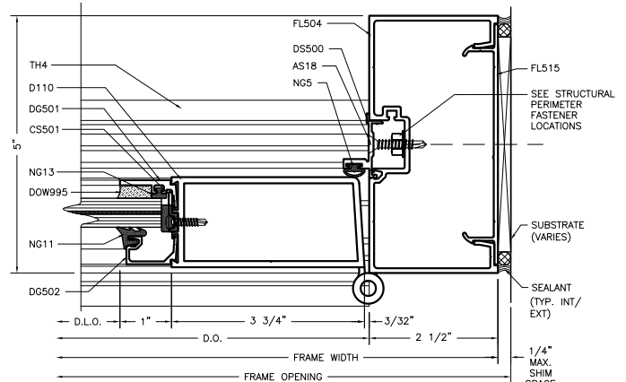
DOOR JAMB AT WALL 1:2
