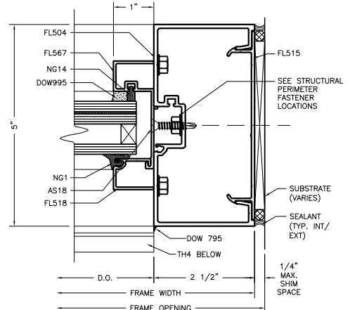
TRANSOM DOOR JAMB AT WALL 1:2
