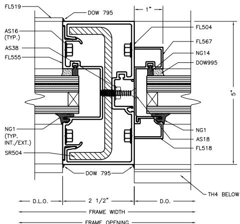
INTERM. DOOR JAMB @ TRANSOM 1:2
