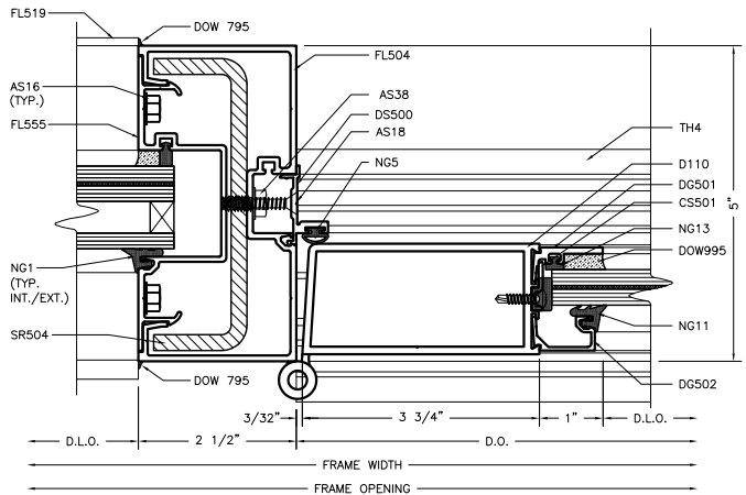
INTERM. DOOR JAMB 1:2
