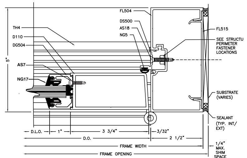
DOOR JAMB AT WALL 1:2
