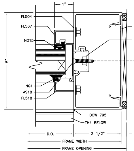
TRANSOM DOOR JAMB AT WALL 1:2
