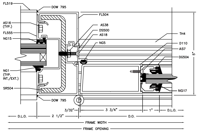
INTERM. DOOR JAMB 1:2
