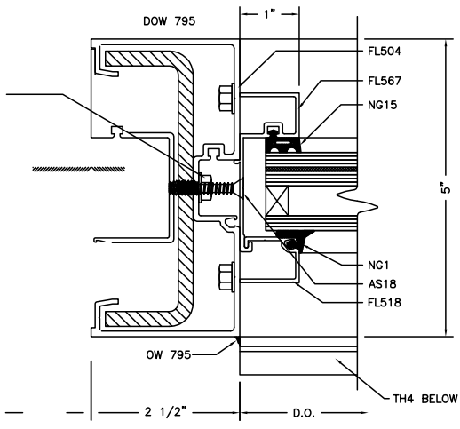
DOOR JAMB @ TRANSOM 1:2
